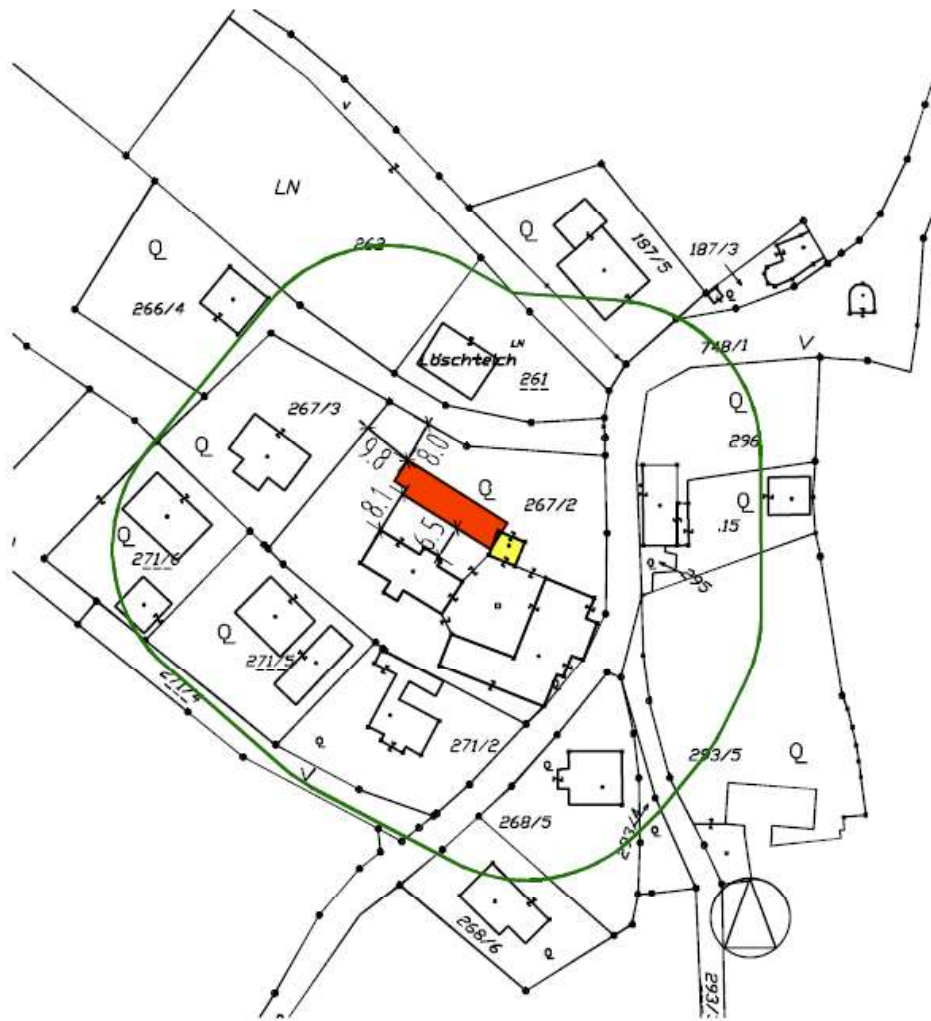
LAGEPLAN 1_1000
