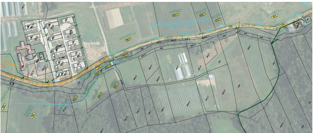
Der Verlauf der neuen Wasserleitung zwischen ZB II und ZB I im Kötschmanngraben
